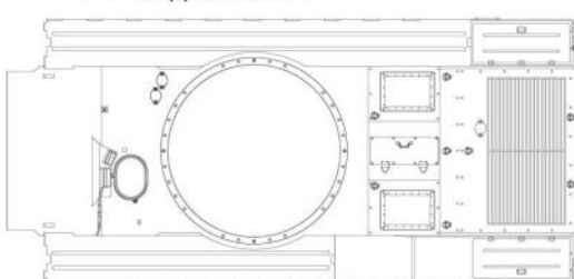
车面 Upper Hull X 1
