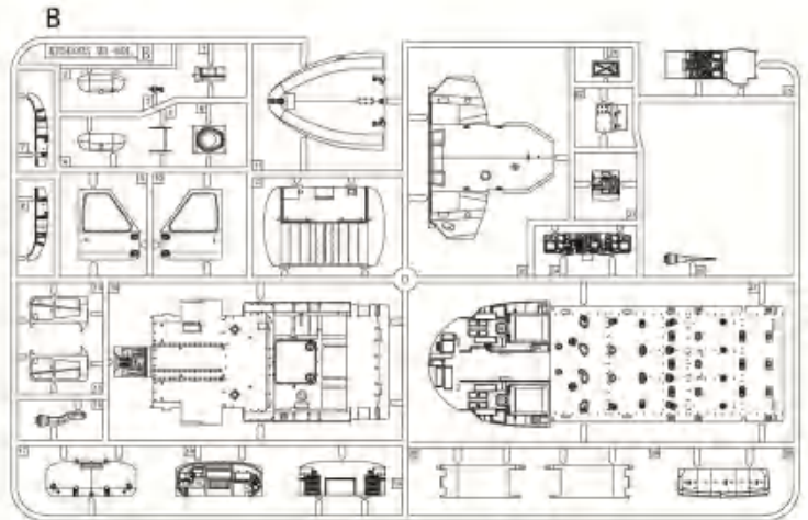
《右側機身》 Right fuselage
